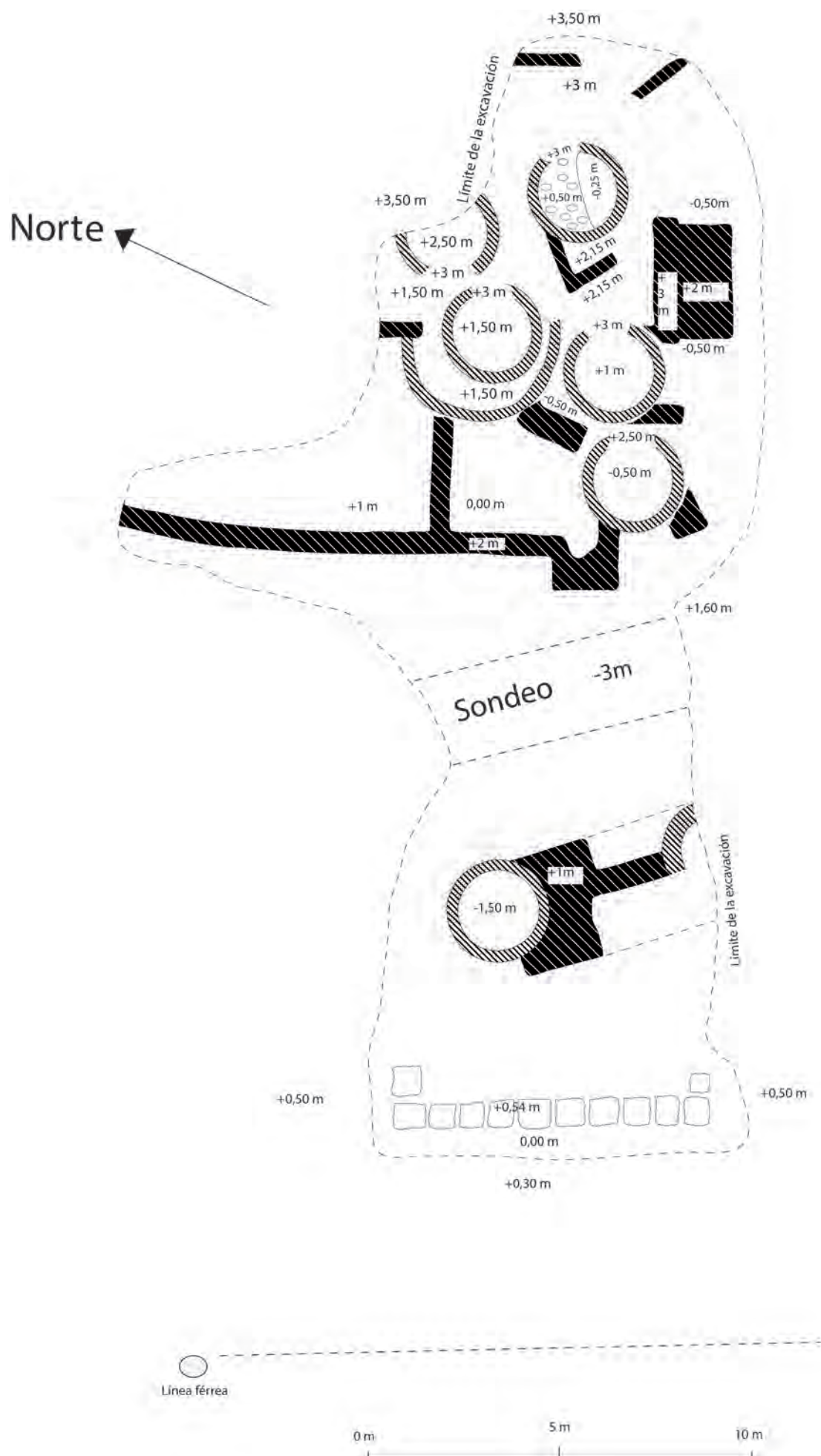
PLANO 20: Calco actualizado del sector de hornos cerámicos descubiertos en un sondeo al Sur del kom en 1928 a partir de BISSON DE LA ROQUE 1933: pl. IV. (Zulema Barahona Mendieta).
