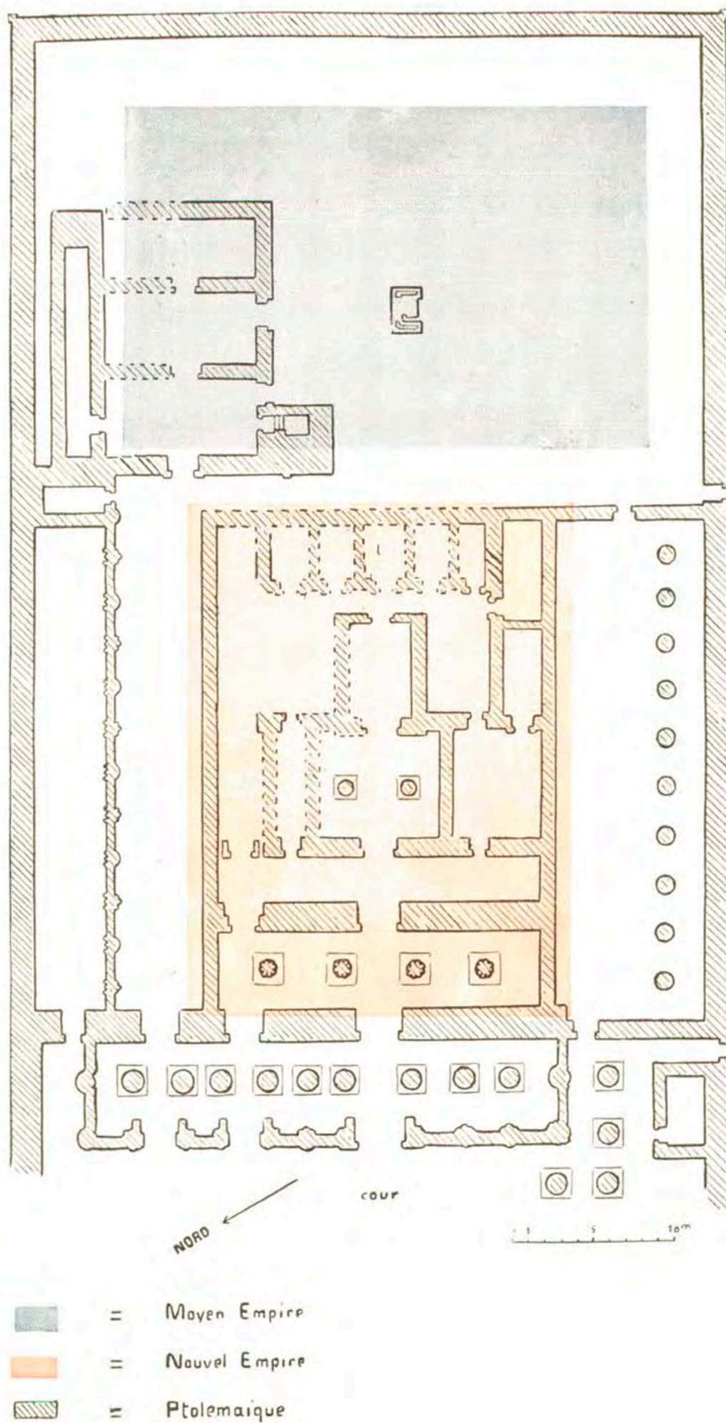
PLANO 10: Plano del templo con la interpretación de las distintas plataformas de cimentación según Bisson de la Roque (BISSEON DE LA ROQUE 1929: pl. II).
