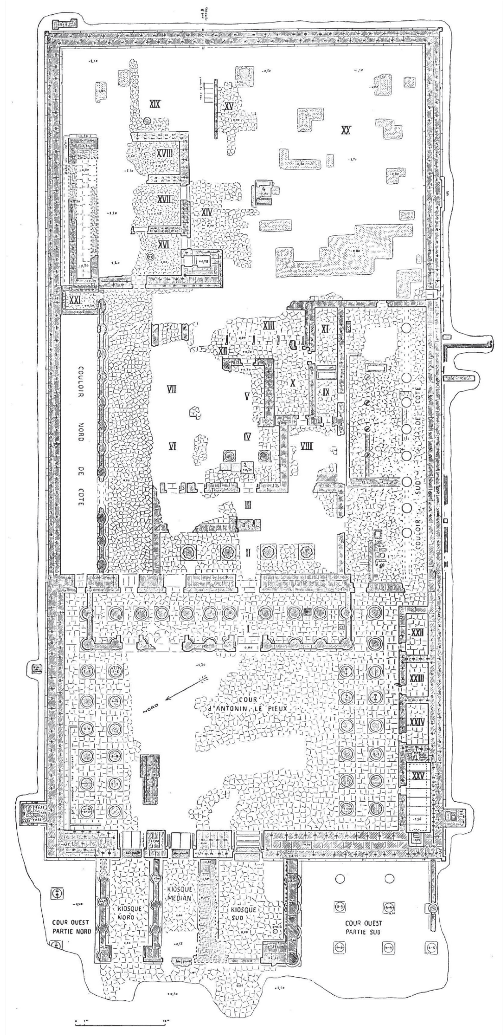
PLANO 4: Plano del templo, con la designación de las divisiones creadas a partir de 1926 (BISSEON DE LA ROQUE 1927: pl. I) .
