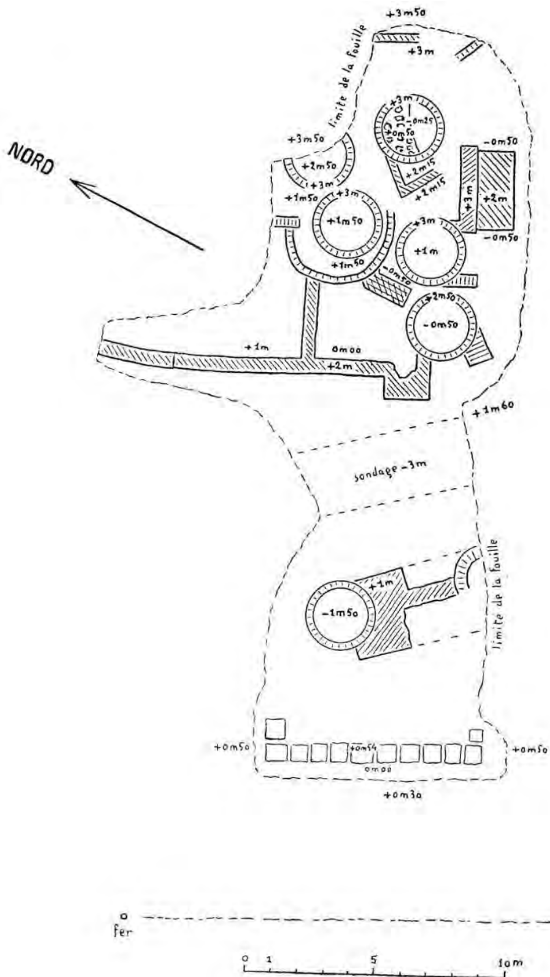
PLANO 19: Plano del sector de hornos cerámicos descubiertos en un sondeo al Sur del kom en 1928 (BISSEON DE LA ROQUE 1933: pl. IV).
